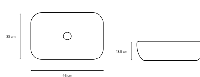
VARI 46 - 46 x 33 x 13,5 cm
